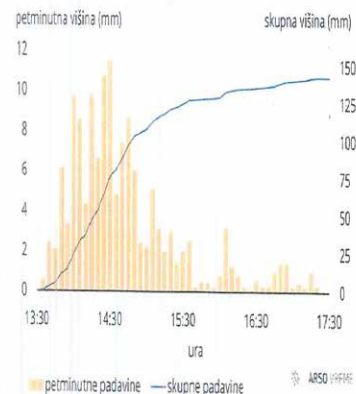
Slika 7. Časovni potek petminutne in skupne višine padavin na Muti pri Dravogradu ob nalivu 24. avgusta popoldne
